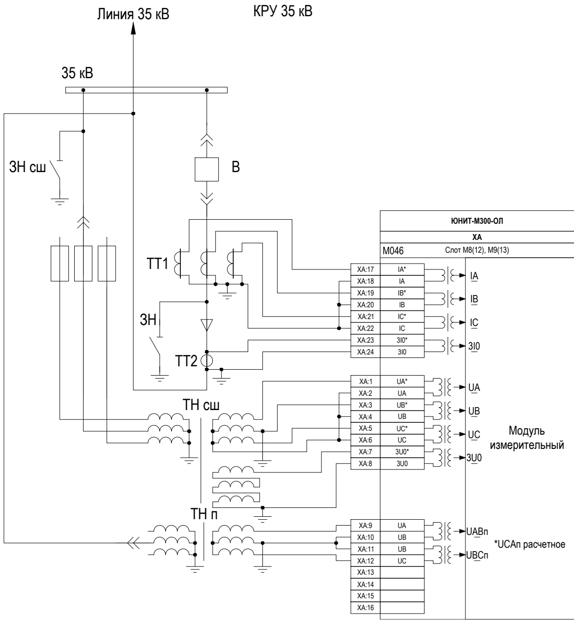
Рисунок Г.2 – Пример подключения аналоговых цепей трансформаторов тока и напряжения для РУ 35 кВ
